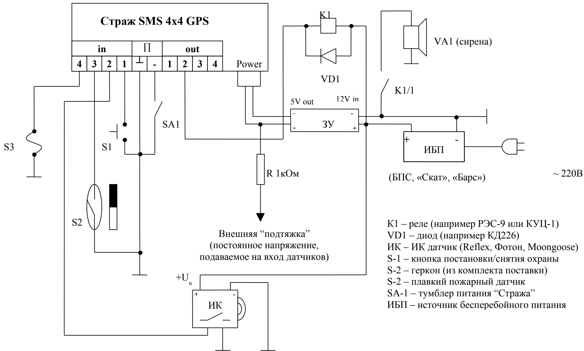
Пример подключения системы «Страж SMS 4x4 GPS» в качестве системы охраны дома
